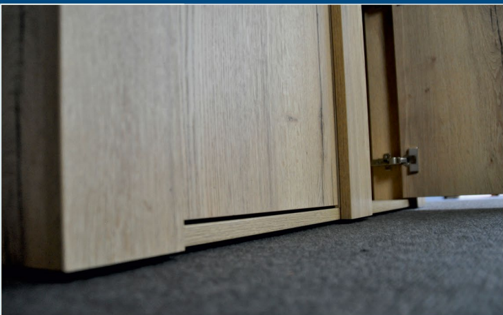
EFS Timber-Line Detail / ohne Sockel - zurückgesetzte Tür
